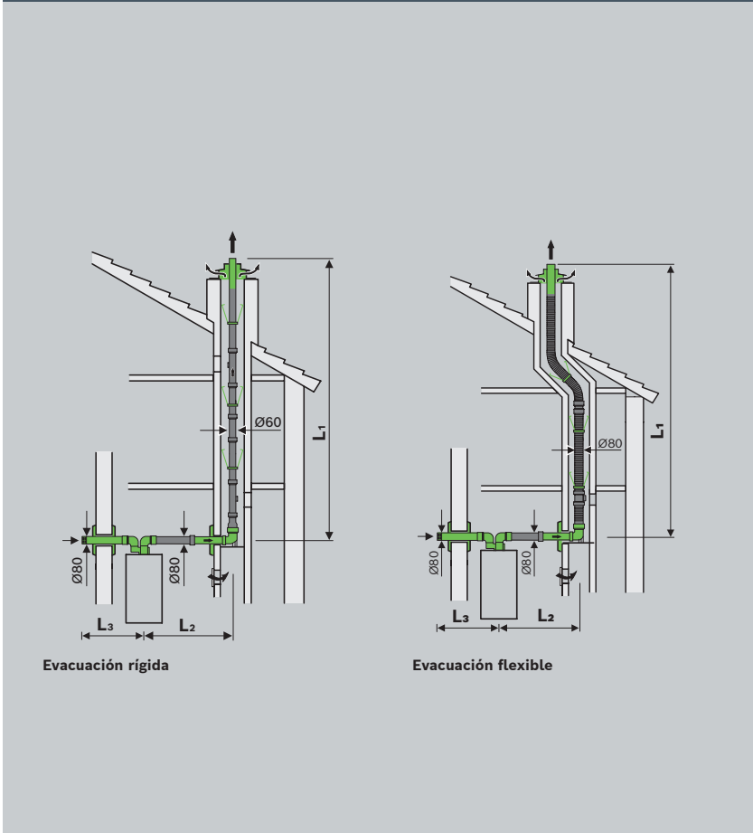
Instalación C53x DN 80
