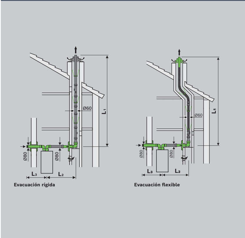
Instalación C53x DN 80
