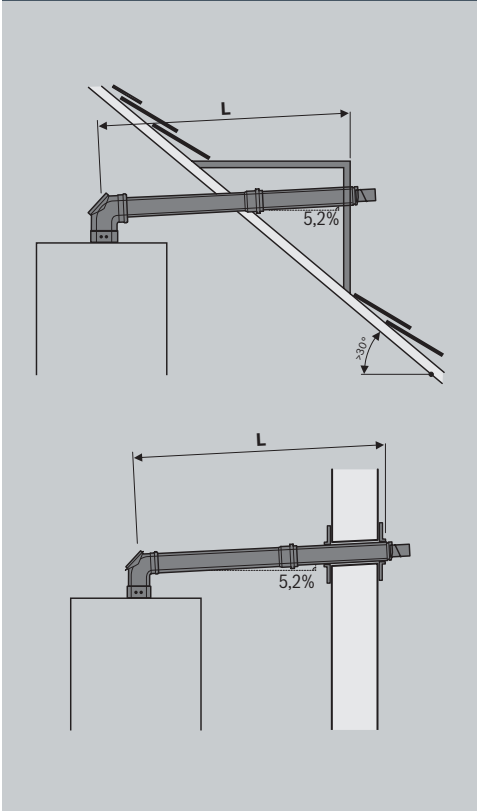
Instalación C33x DN 60/100 y 80/125
