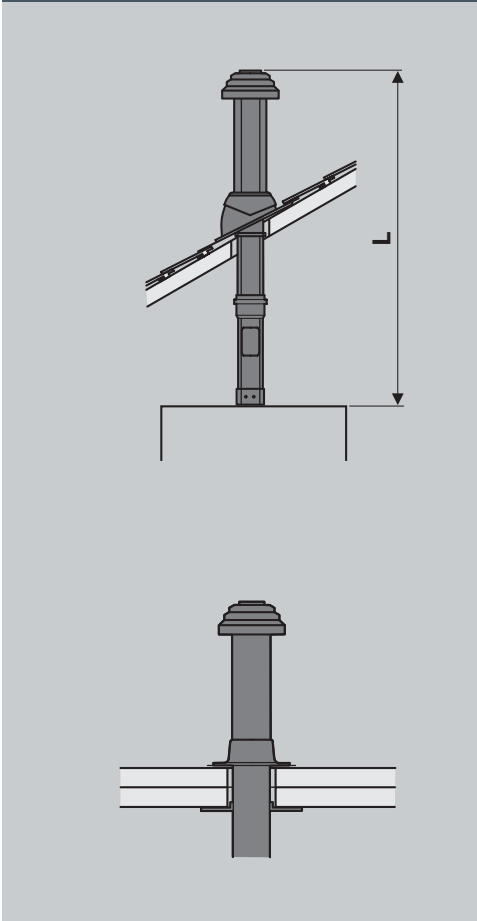
Instalación C33x DN 60/100 y 80/125
